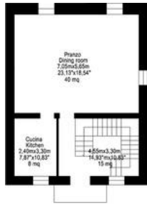
8 ABITAZIONE CASARO PIANO PRIMO FIRST FLOOR
